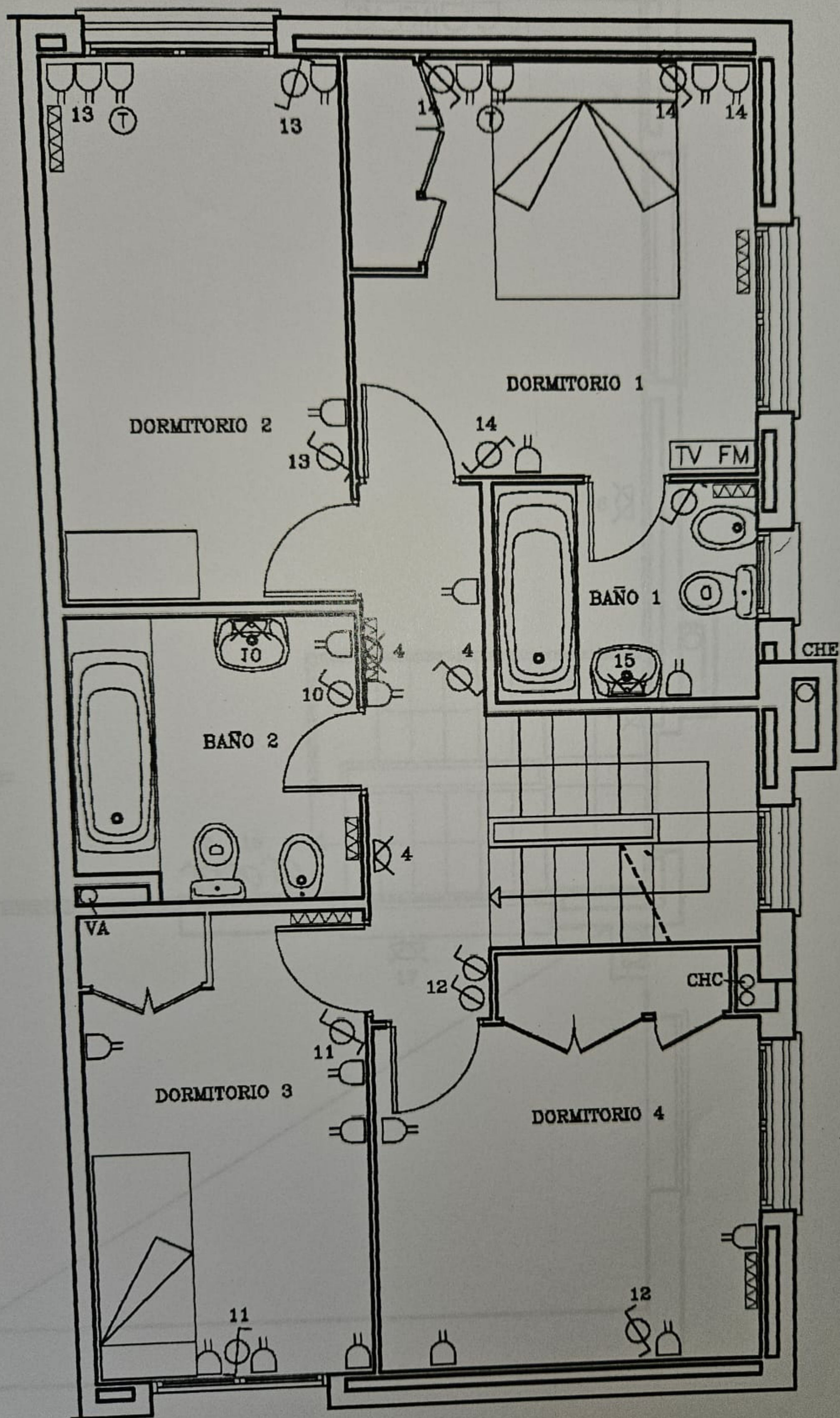
CASA 10B PLANTA PISO
