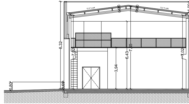
SECCIO B-B'
