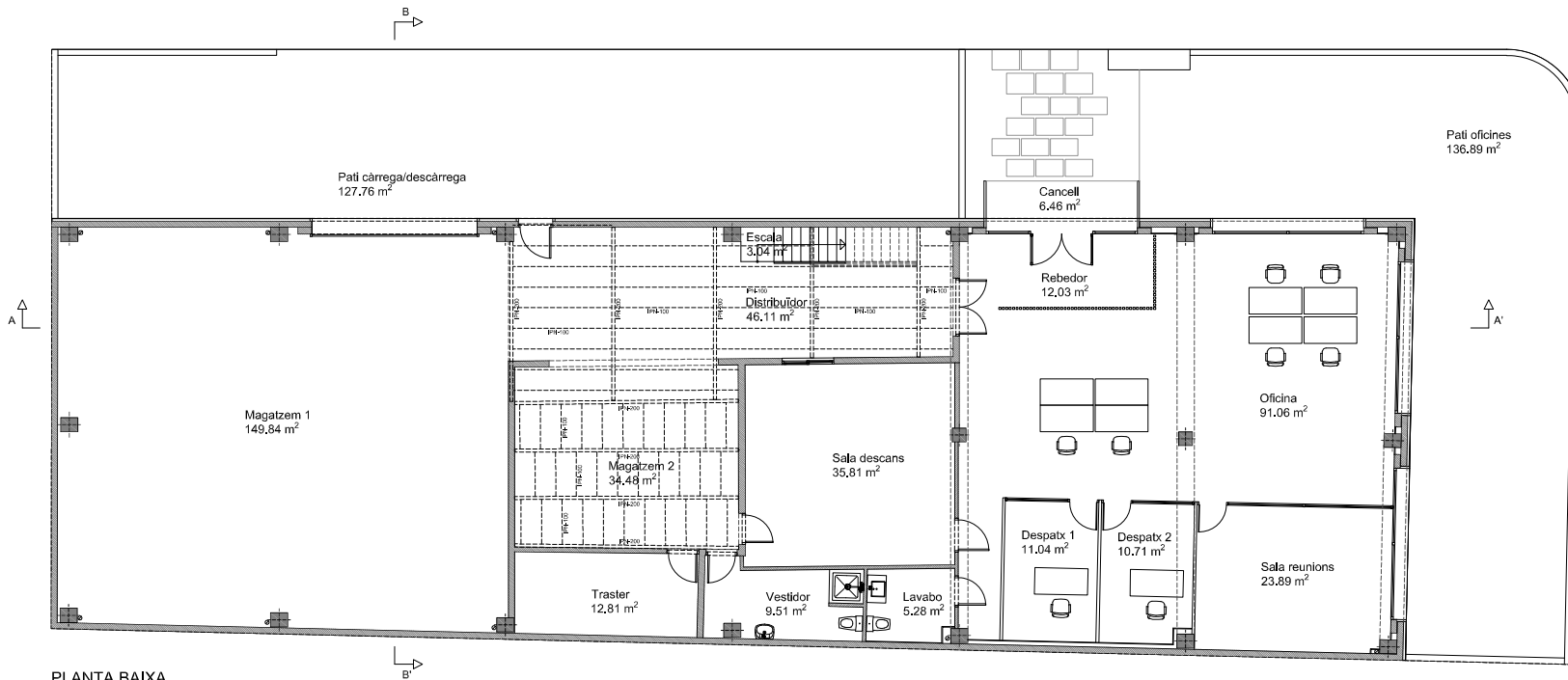
PLANTA BAIXA
