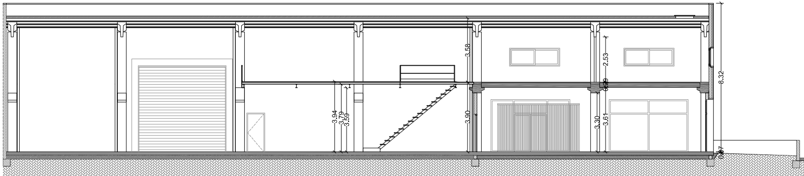
SECCIO A-A'
